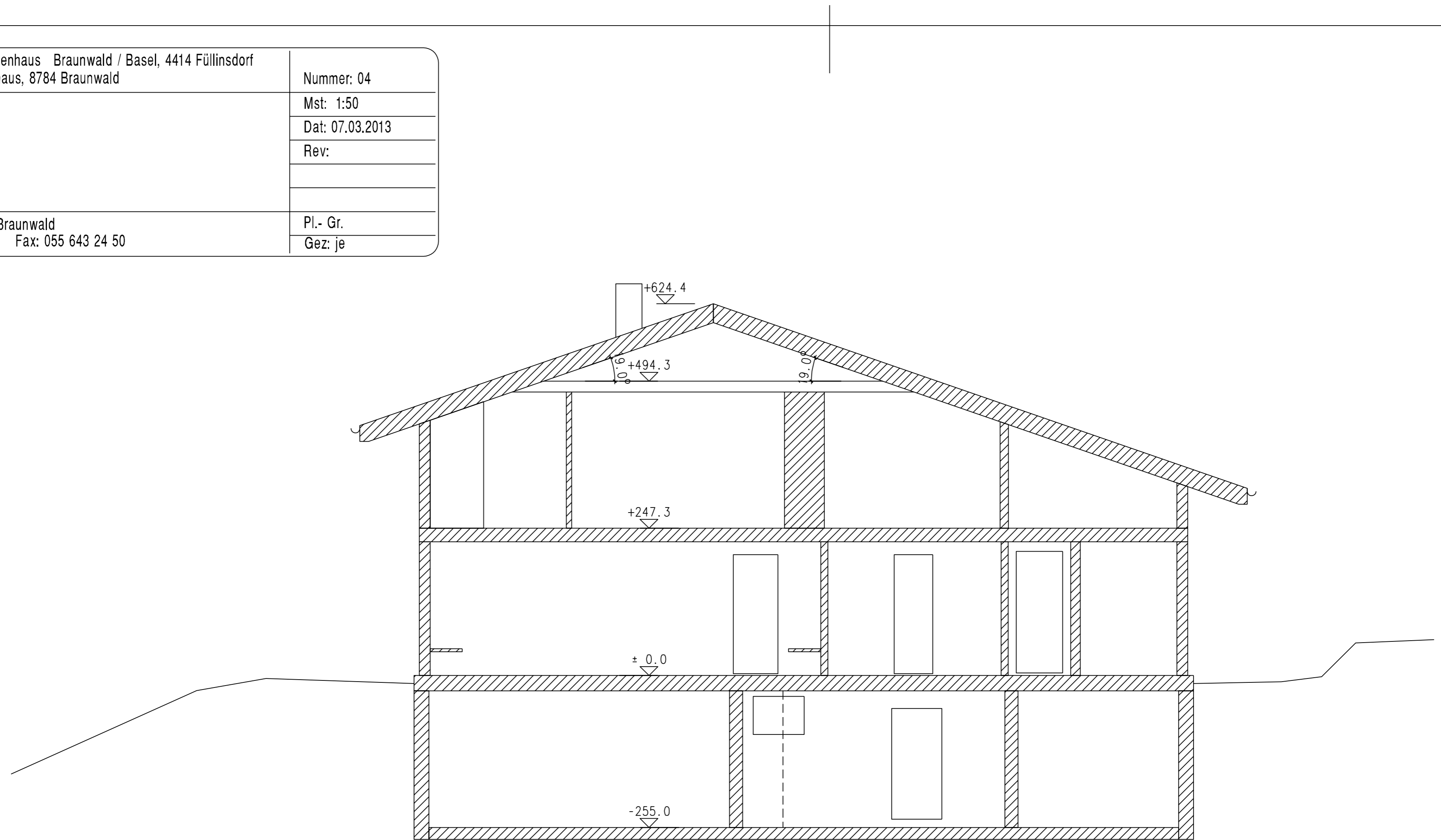
Querschnitt Mst: 1:50
